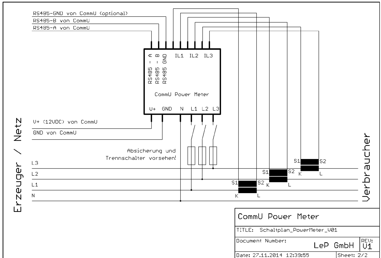
Abbildung 8: Anschlussbild
